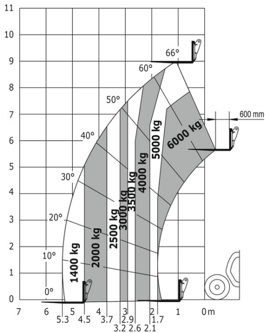
Industrial load chart (EN 1459 A) Metric
